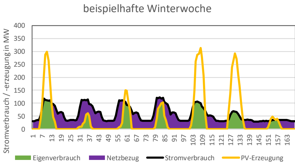
Abbildung 1-1: Lastgang und Erzeugung in einer beispielhaften Winterwoche mit Schulbetrieb
