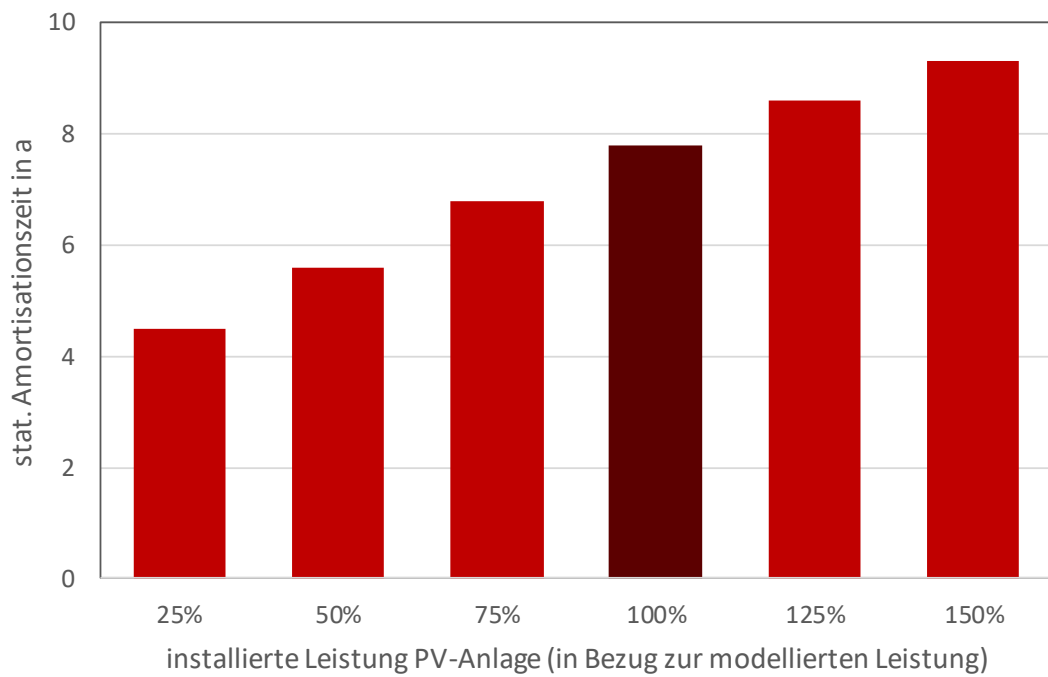
Abbildung 1-5: Variierte installierte PV-Leistung von 25 % bis 150 % zur Berechnung der Amortisation
