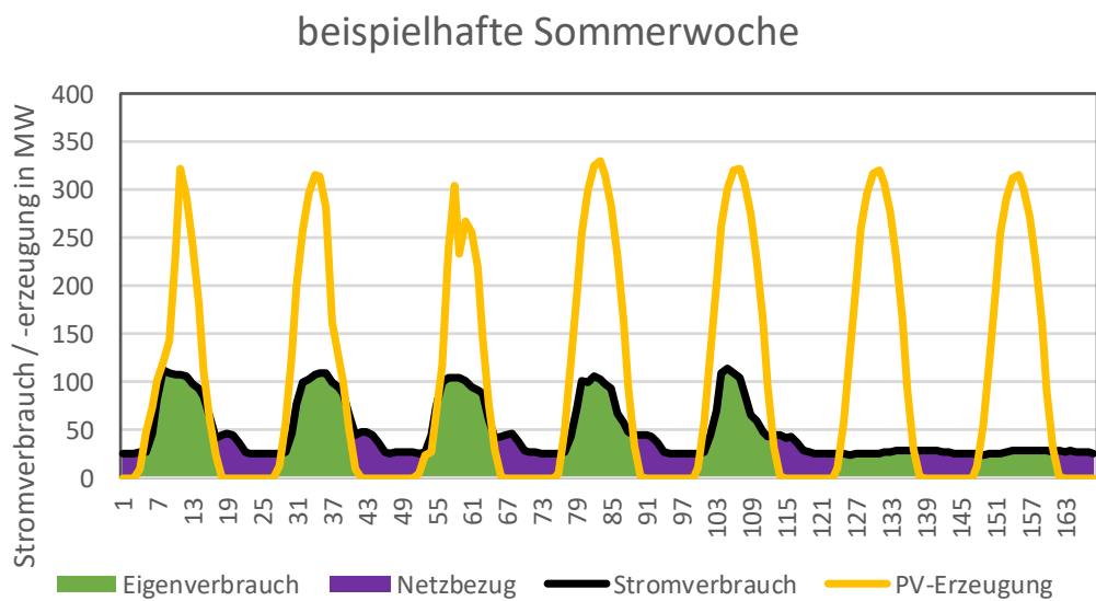
Abbildung 1-2: Lastgang und Erzeugung in einer beispielhaften Sommerwoche mit Schulbetrieb
